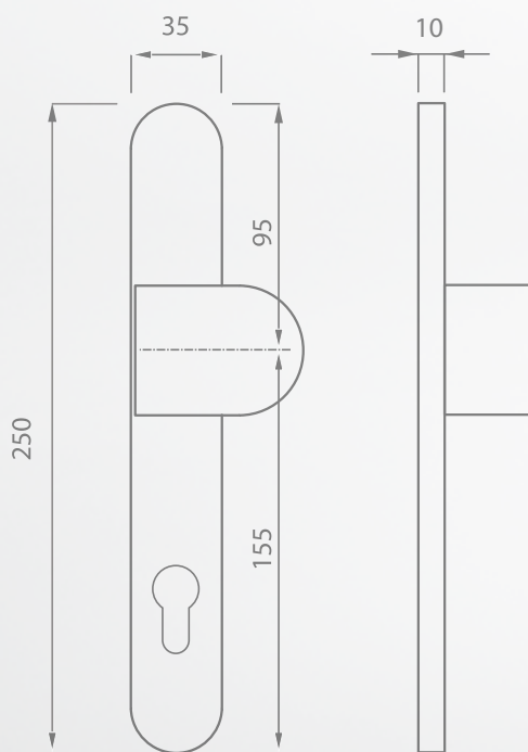
Vnější štít
