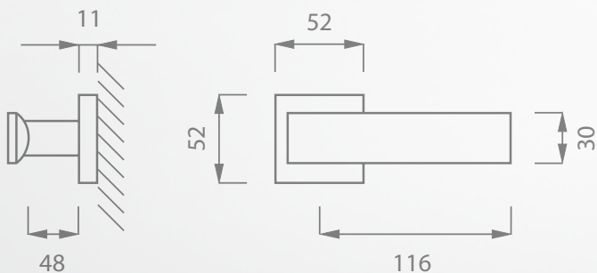
klika
