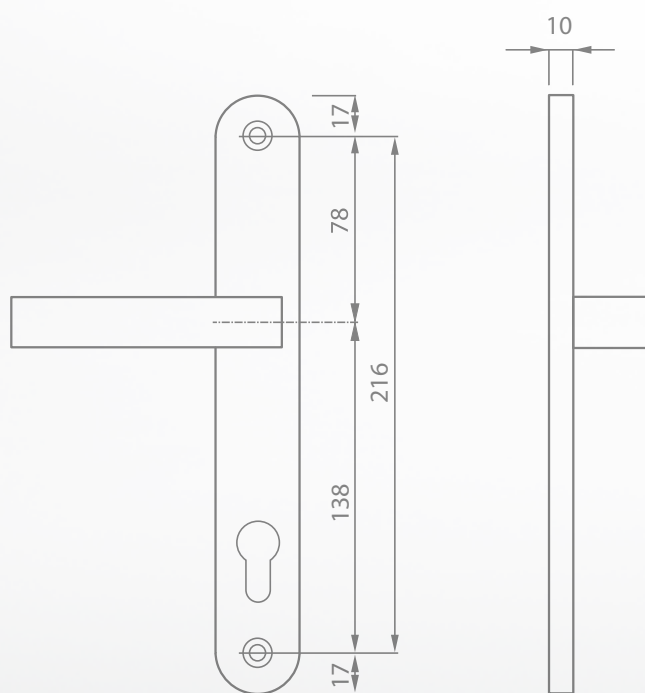
Vnitřní štít
