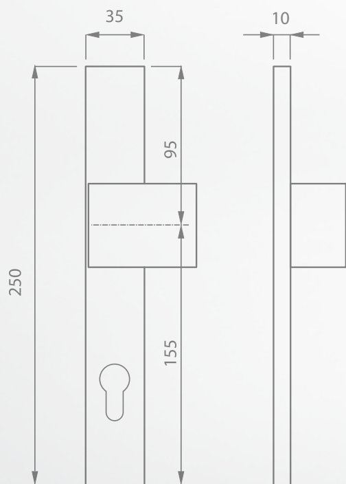
Vnější štít
