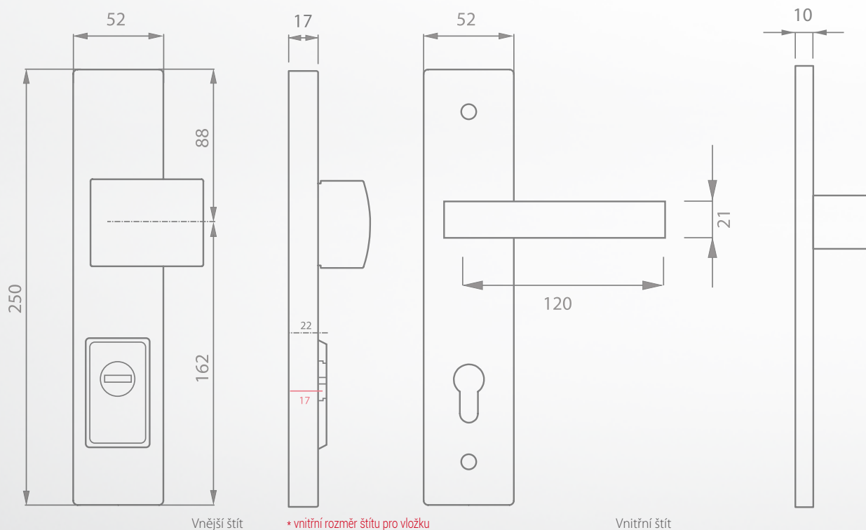
Vnější štít
