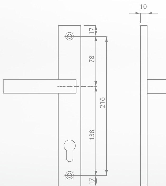
Vnitřní štít
