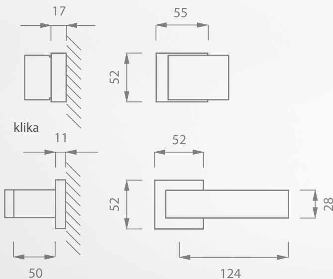
madlo
