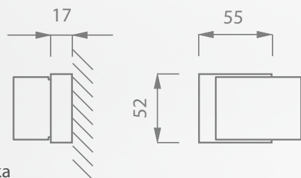
madlo
